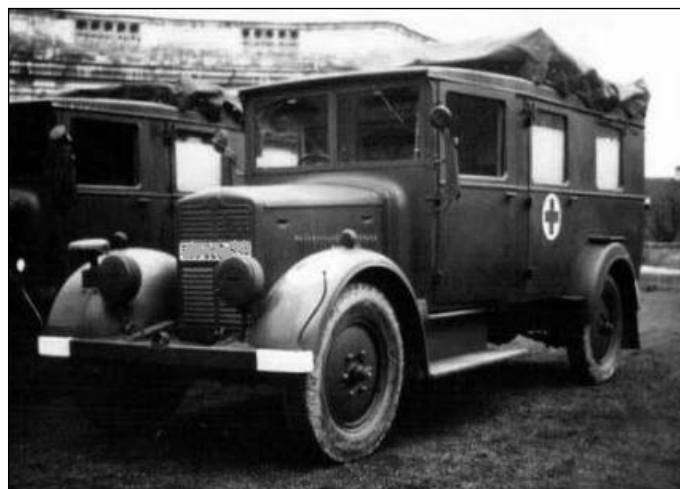
Lehký nákladní automobil Phanomen Granit 25, sanitní verze
