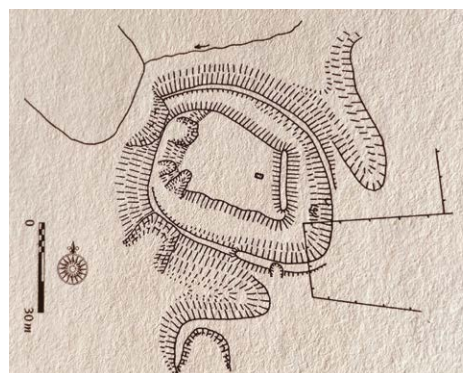
Velké Popovice (Praha-východ), náčrt tvrzíště. Stav rok 1985, záměření T. Tomíček a J. Úlovec, kresba T. Tomíček
