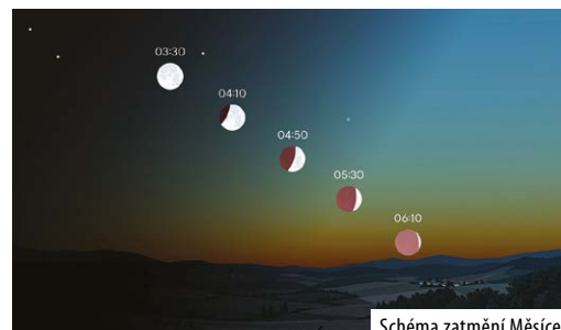
Schéma zatmění Měsíce
