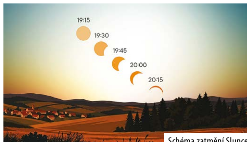
Schéma zatmění Slunce
